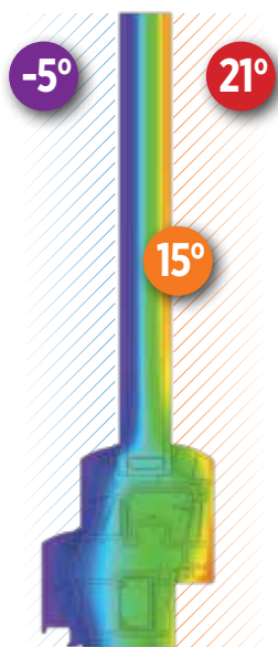
PVC RAAM 72 mm Dubbele beglazing
