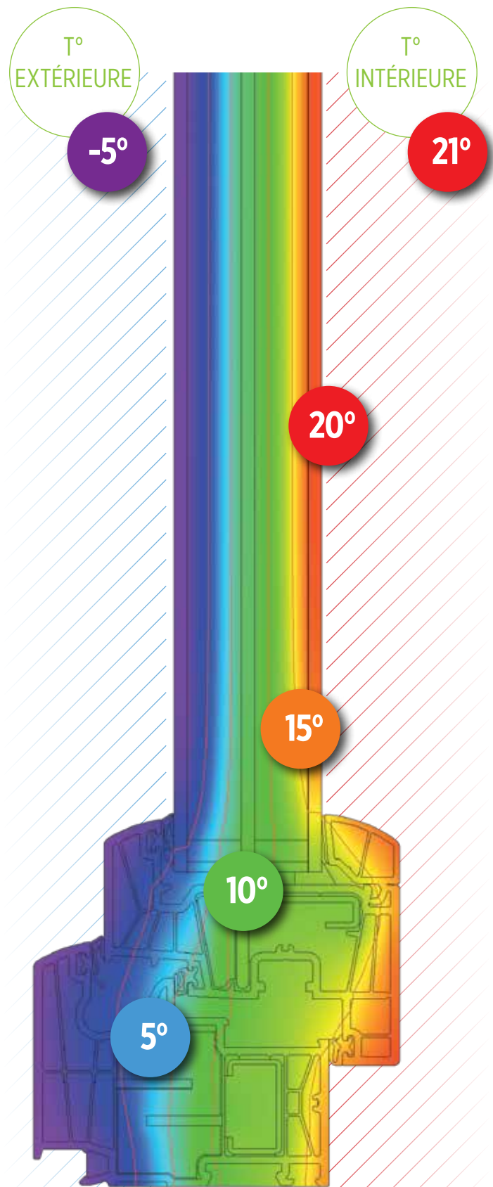
PVC RAAM VAN PIERRET 88 mm Drievoudige beglazing
