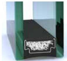
Thermix afstandshouder
